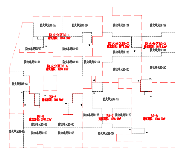
负二层防火分区示意图 1:1000
