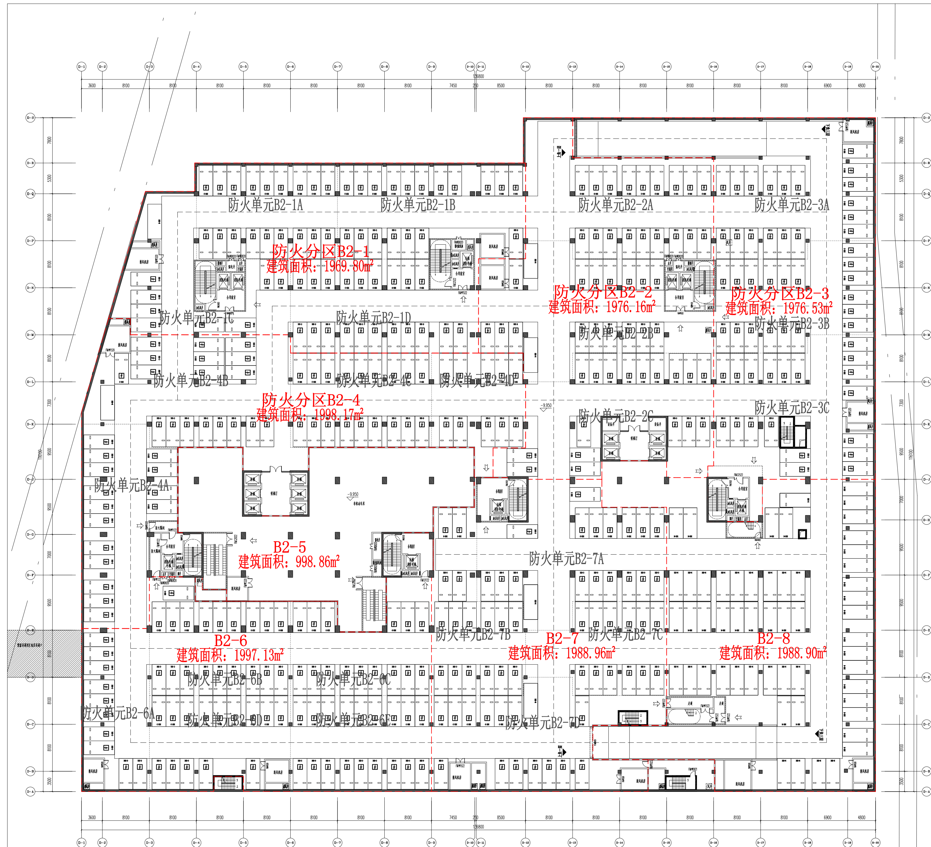
负二层平面图 1:200
