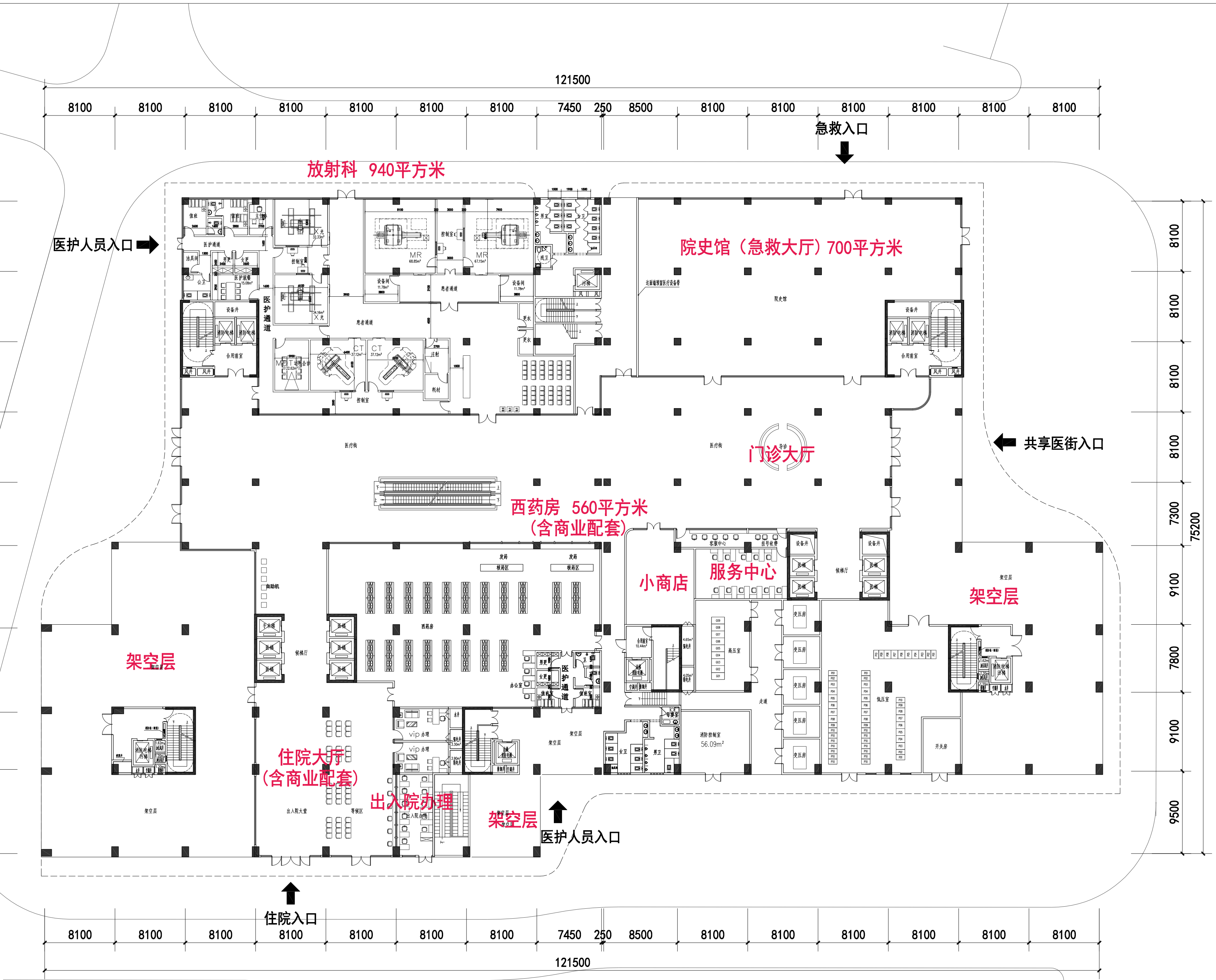
首层平面图
